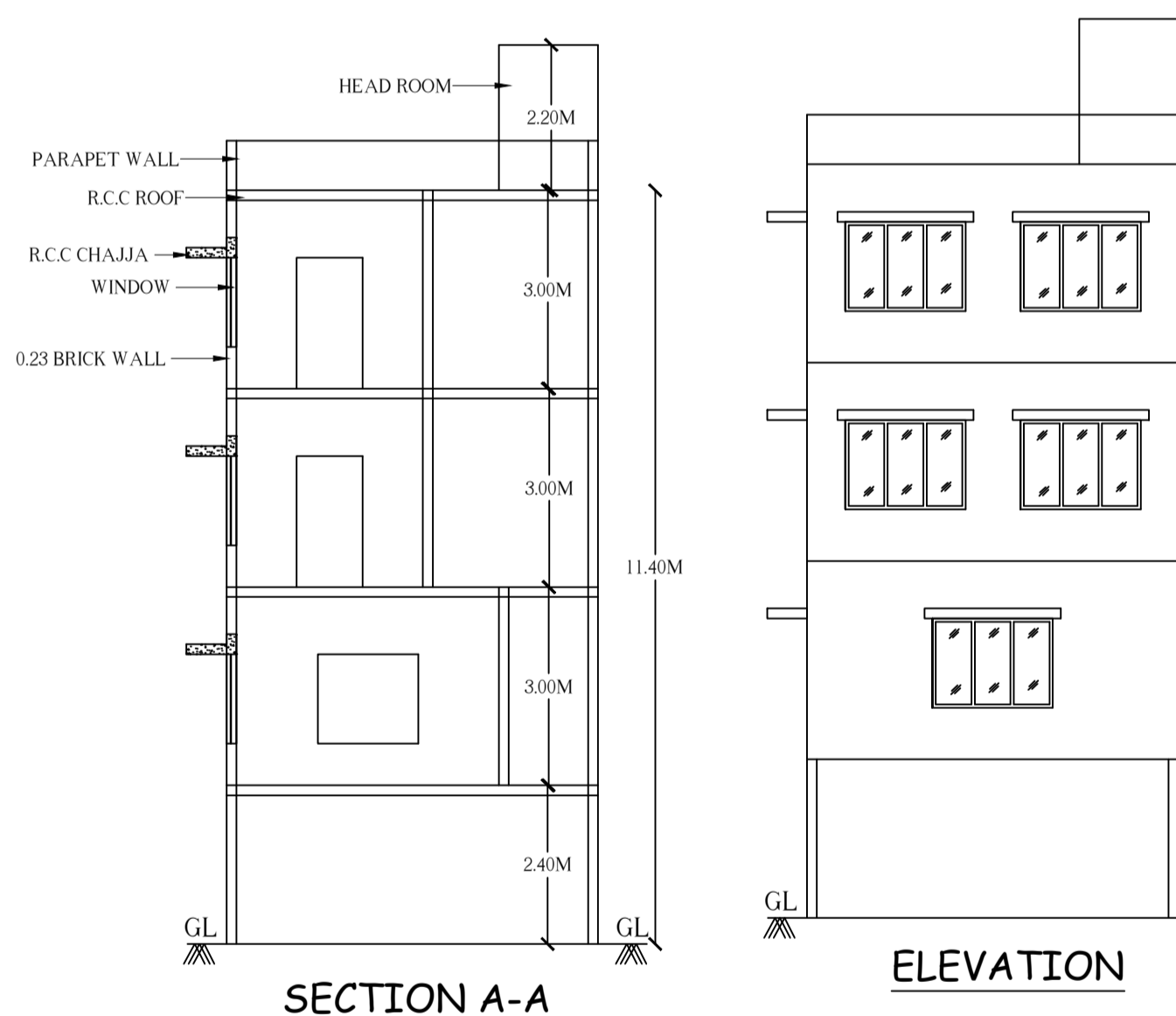
SECTION A-A
